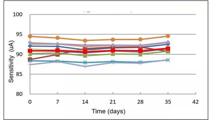
灵敏度漂移 @ 温度 45°C, 湿度 90%
