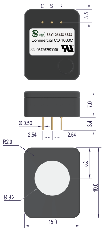
所有尺寸标注以毫米为单位 除非另有说明, 所有公差 \pm 0.20 毫米
